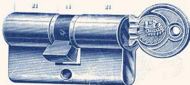
240. Cylindr 53 m. m. dl. pro dvoukřídlové dveře Zylinder 53 m. m. lang für Zweiflügeltür.
