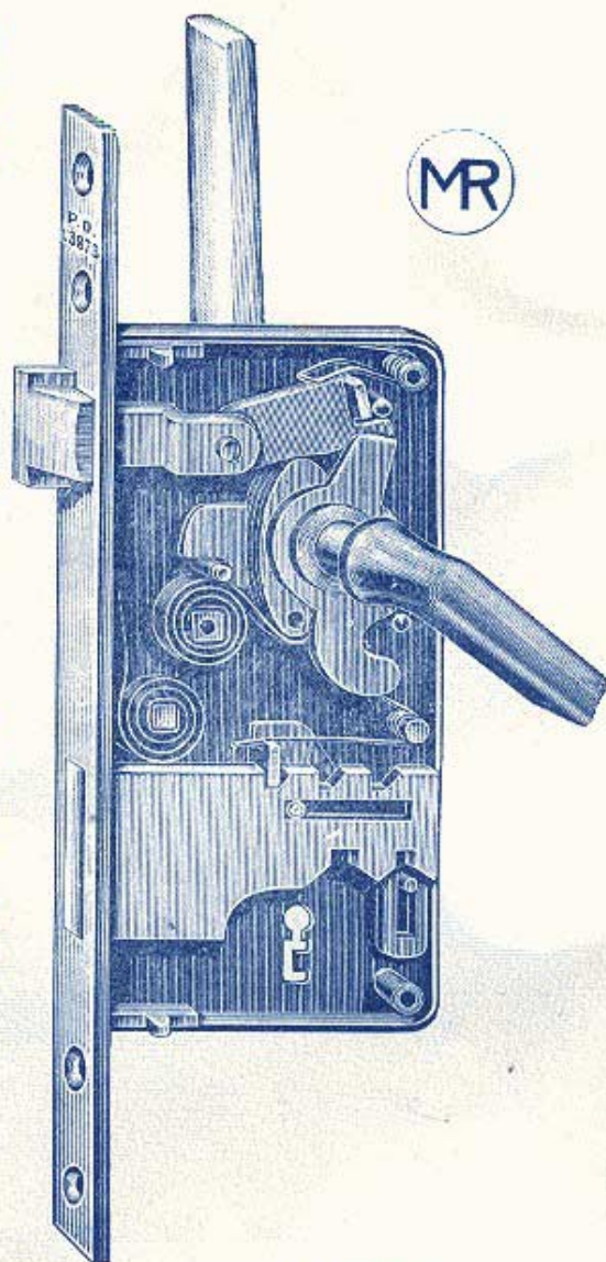
Vyobrazení II. Poloviční velikost.
