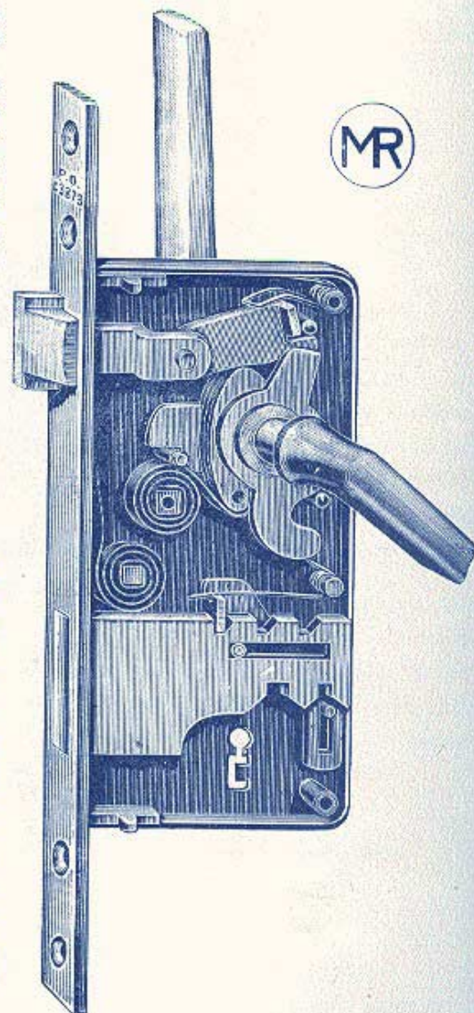
Abbildung II. Halbe natürliche Grösse
