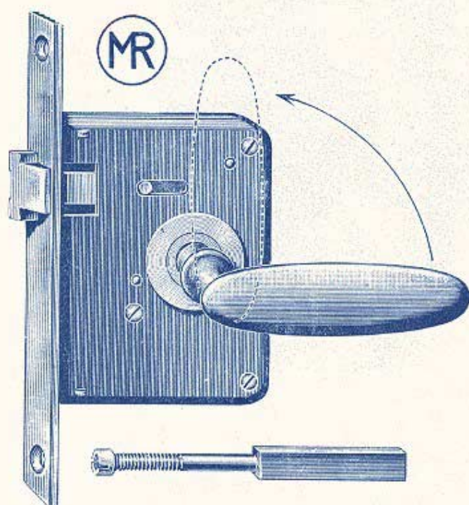
Čep pro blokovací kliky.
