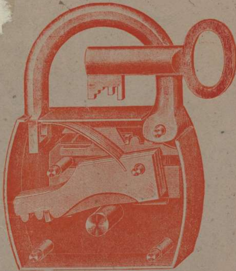
Ukázka vnitřního zařízení zámku „Custos“ velikosti 775 E.
